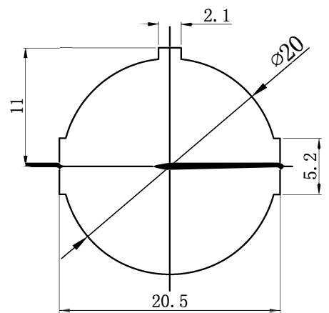
安装面板尺寸 PANEL CUT-OUT
